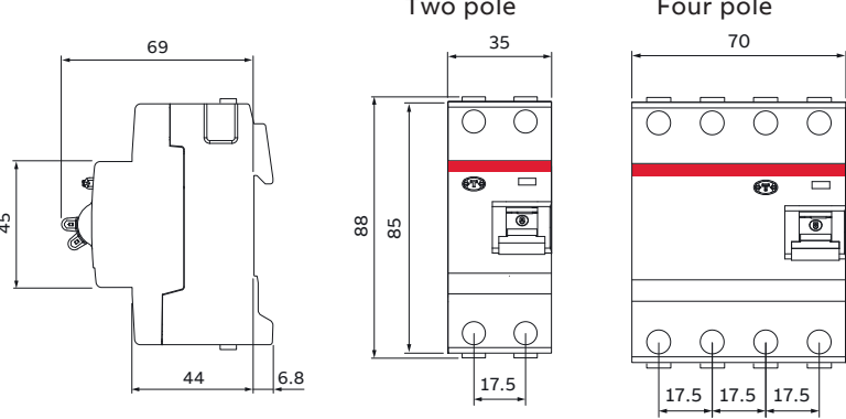
RCCB F200
